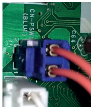
Złącze presostatu HP CN-PSW1
