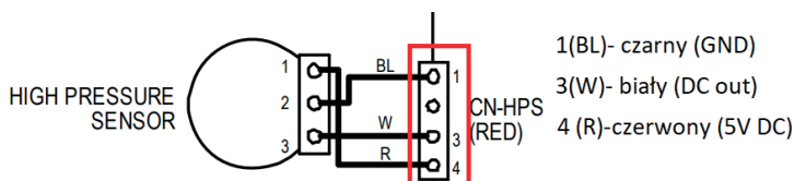
Złącze przetwornika HP CN-HPS
